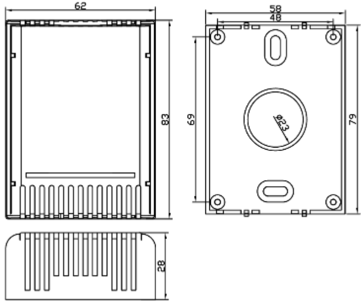
그림1 AW-M30R 제품 치수
