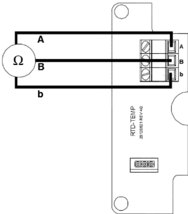
그림2 전기 결선도
